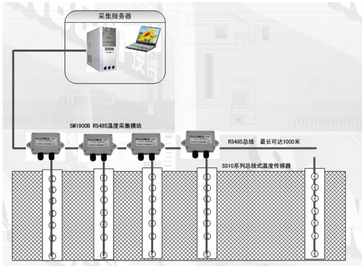
图 1.1 测温原理示意图
